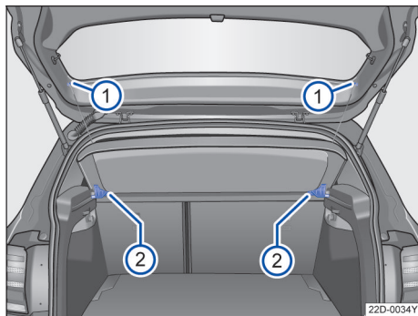
图 128 拆卸和安装行李厢盖板
