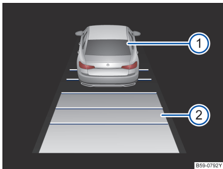
图 103 组合仪表显示屏：已暂时关闭自适应巡航系统（ACC）控制功能，已探测到的前方车辆，设定的距离间隔
