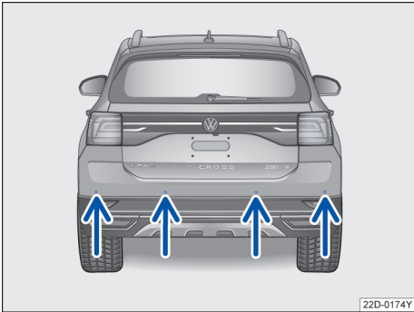
图 114 后部泊车雷达探头位置
