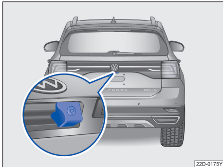
图 117 车辆行李厢盖内：倒车摄像头的安装位置
