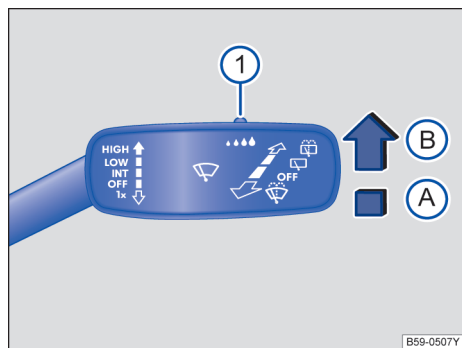
图 78 车窗玻璃刮水器操作杆：调节雨量传感器 ①
