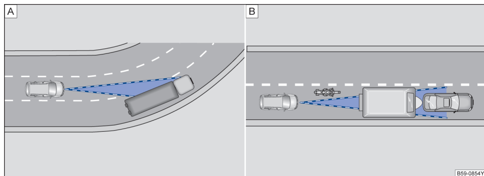
图 107 A. 处在弯道里的汽车 B. 前方行驶的摩托车处在雷达传感器探测范围外
