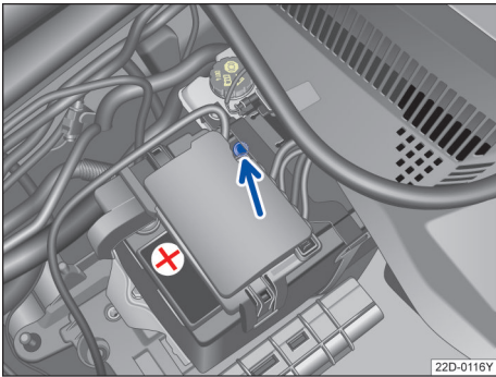
图 159 蓄电池电眼
