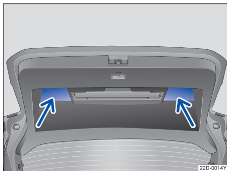
图 55 已打开的行李厢盖：用于关上的凹槽
