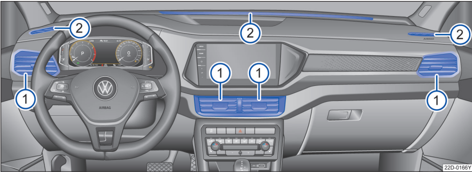
图 88 前部通风口
