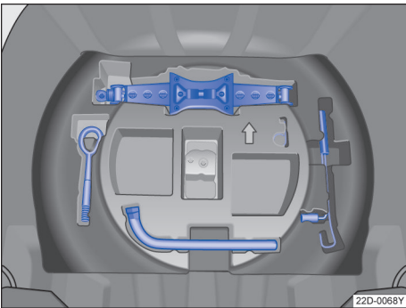
图 137 行李厢垫下的随车工具
