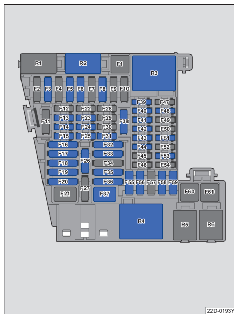
图 144 仪表板中：保险丝位置示意图
