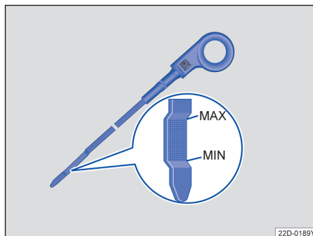
图 155 带液位标记的机油标尺
