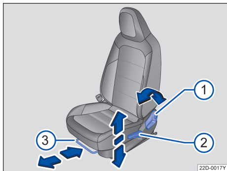
图 61 手动调整式座椅上的操作元件
